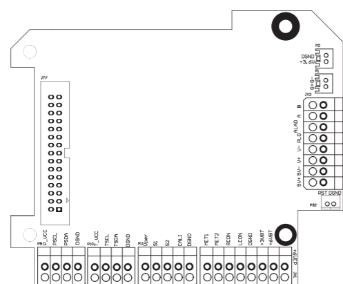
图16 接线接口和按键排列图
