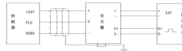
图19 脉冲输出（可选安全栅GS8052）
