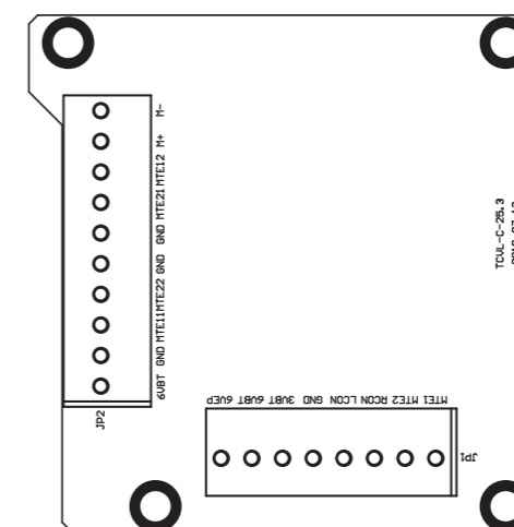
图18 阀门控制板接线接口
