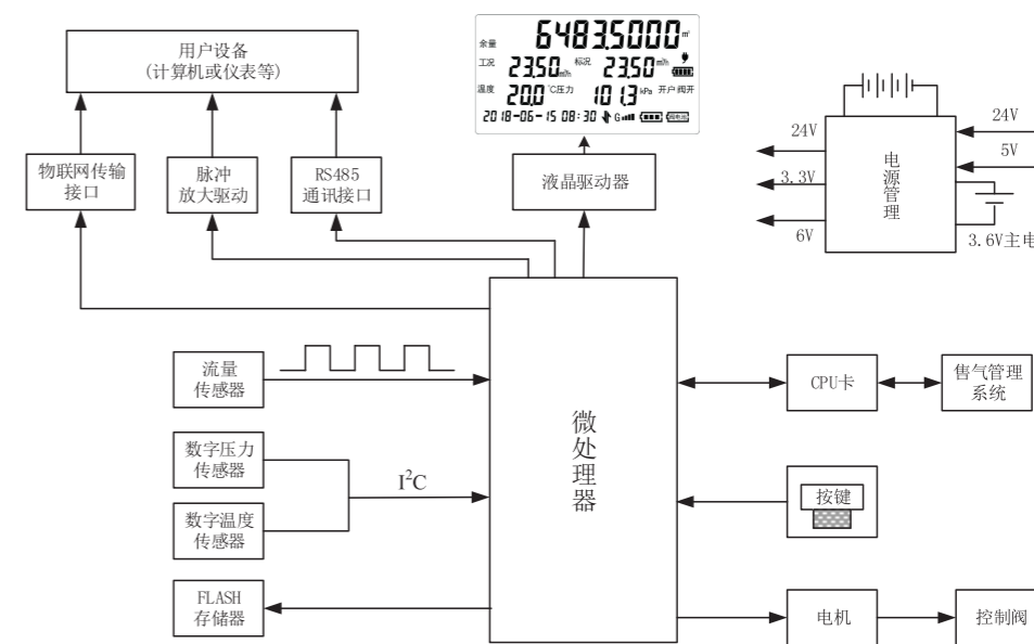
图1 CPU卡流量补偿控制仪原理框图
