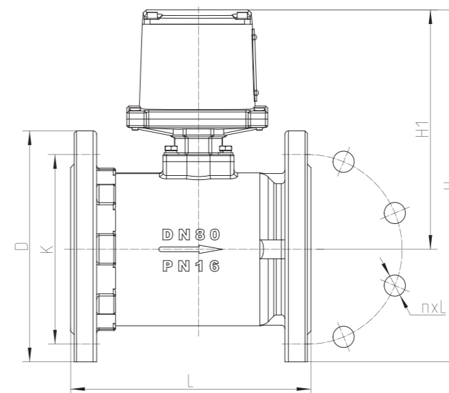
图2 外形图
