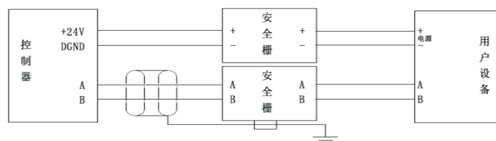
图20 RS485通信 (可选安全栅GS8093B)
