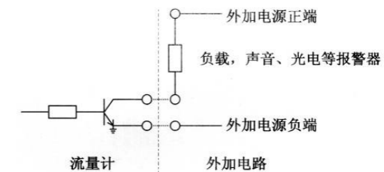
图13 报警电路图
