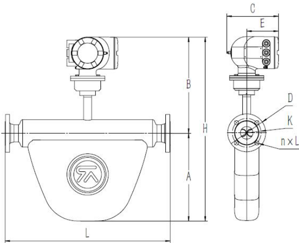
一体式尺寸图
