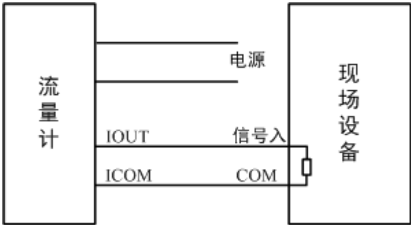
图 5 电流输出
