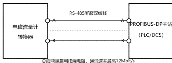
图 3 PROFIBUS-DP 通讯
