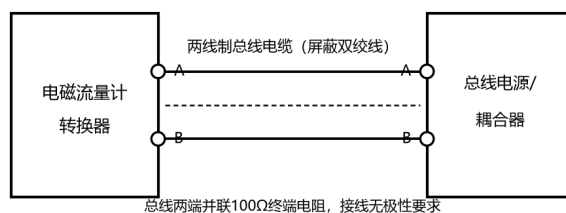
图 2 FF/PROFIBUS-PA 总线通讯
