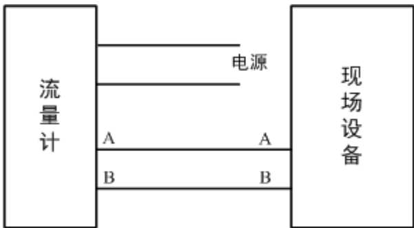
图 1 RS-485 通讯
