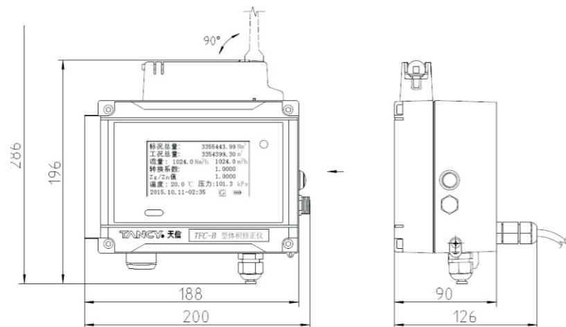
图2 TFC-B外型尺寸图
