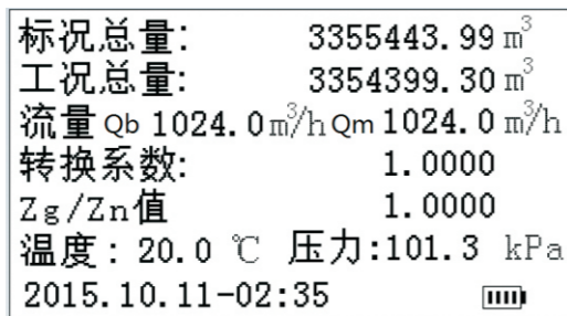
图3 正常运行时修正仪显示
