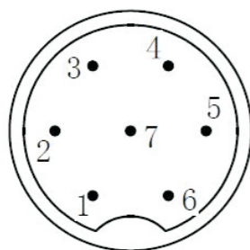
图7 航空插座
