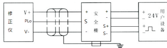
图10 脉冲信号输出 (安全栅可选GS8052)
