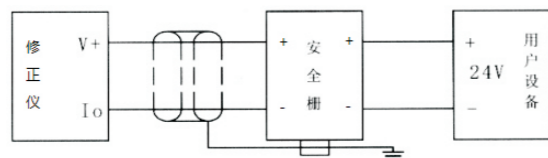
图14 两线制4mA~20mA输出 (安全栅可选GS8047)
