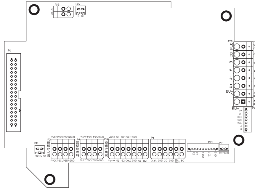
图6 TFC-B接线图
