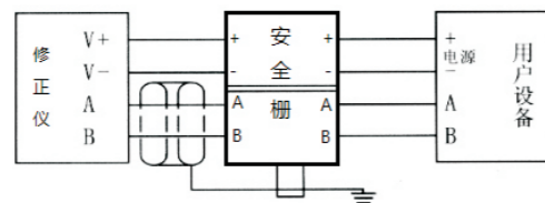
图13 RS485通信接线 (安全栅可选GS8093)
