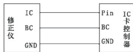
图12 定标脉部信号输出接线
