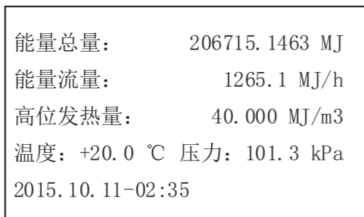
图4 正常运行时修正仪显示 (能量计量版本适用)
