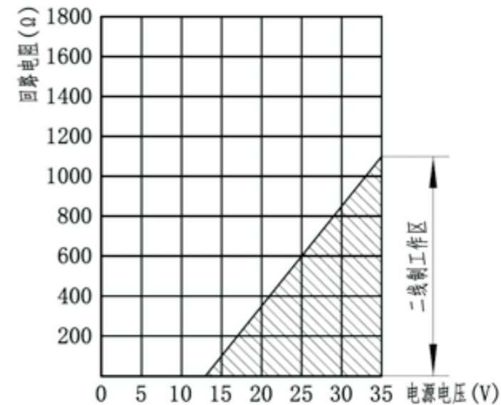
图15 电源电压与回路电阻关系图
