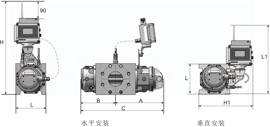
图5-5 G□/TFC-V
