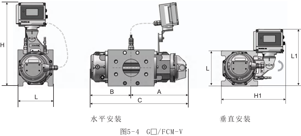
图5-4 G□/FCM-V
