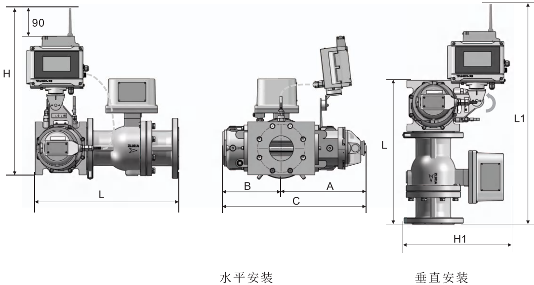
图5-9 G□/TFC-□/TCVL-M-□-R
