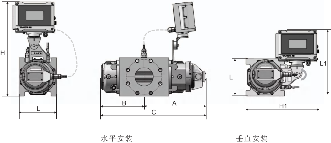
图5-2 G□/FCM
