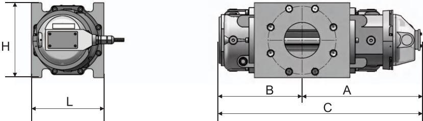
图5-1 G□ 基本型
