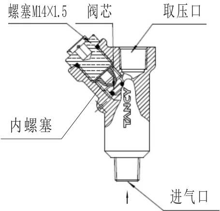
图11 三通保护阀
