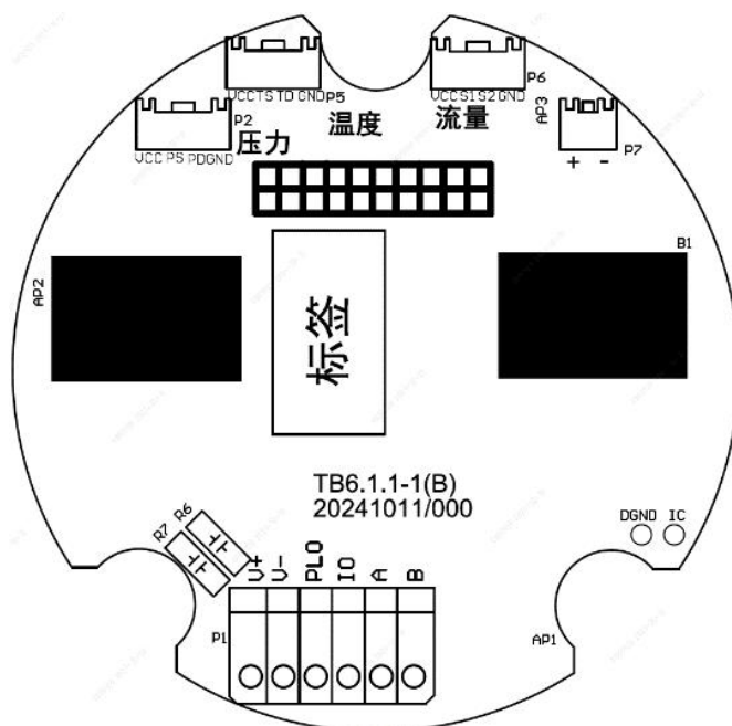
图 7 修正仪接线图
