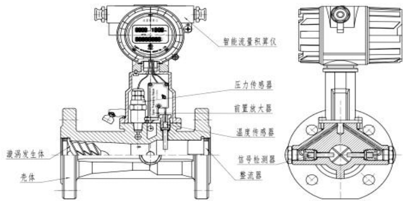
图 1 流量计结构原理图
