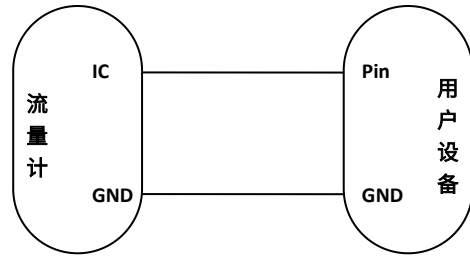
图 8-2 定标脉冲信号输出接线图
