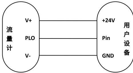
图 8-1 脉冲信号输出接线图
