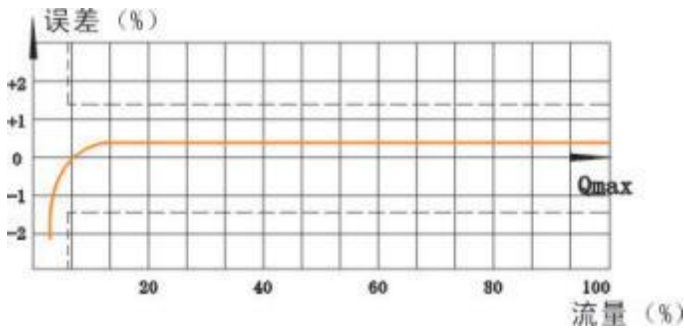
图 2 典型误差曲线图
