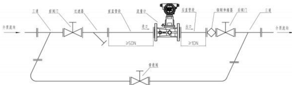
图 4-3 流量计水平安装示意图
