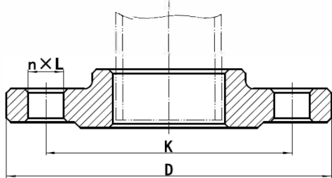
图4-5 突面（RF）带颈平焊钢制管法兰
