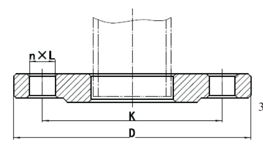
图4-3 突面 (RF) 板式平焊钢制管法兰
