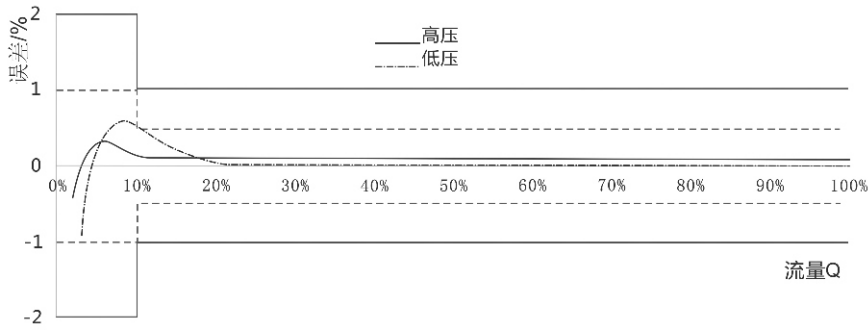
图2 典型误差曲线图
