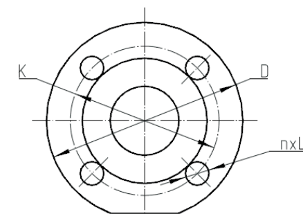
图4-1 法兰连接尺寸图
