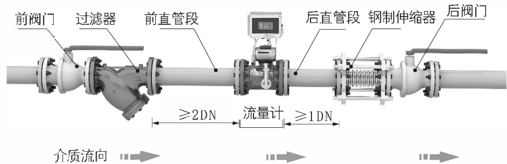
图5 流量计水平安装示意图
