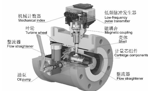
图1 流量计结构原理图
