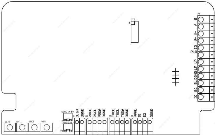
图 7 接线图
