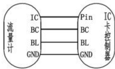
图 12-2 定标脉冲信号输出接线图
