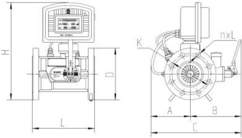
图 5 流量计外形图
