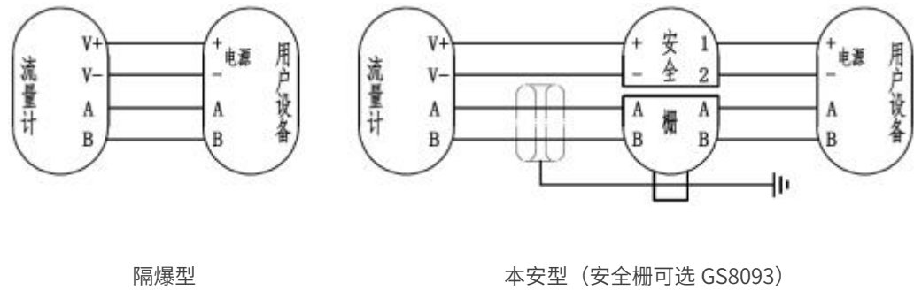
图 12-3 RS485 数据通讯接线图
