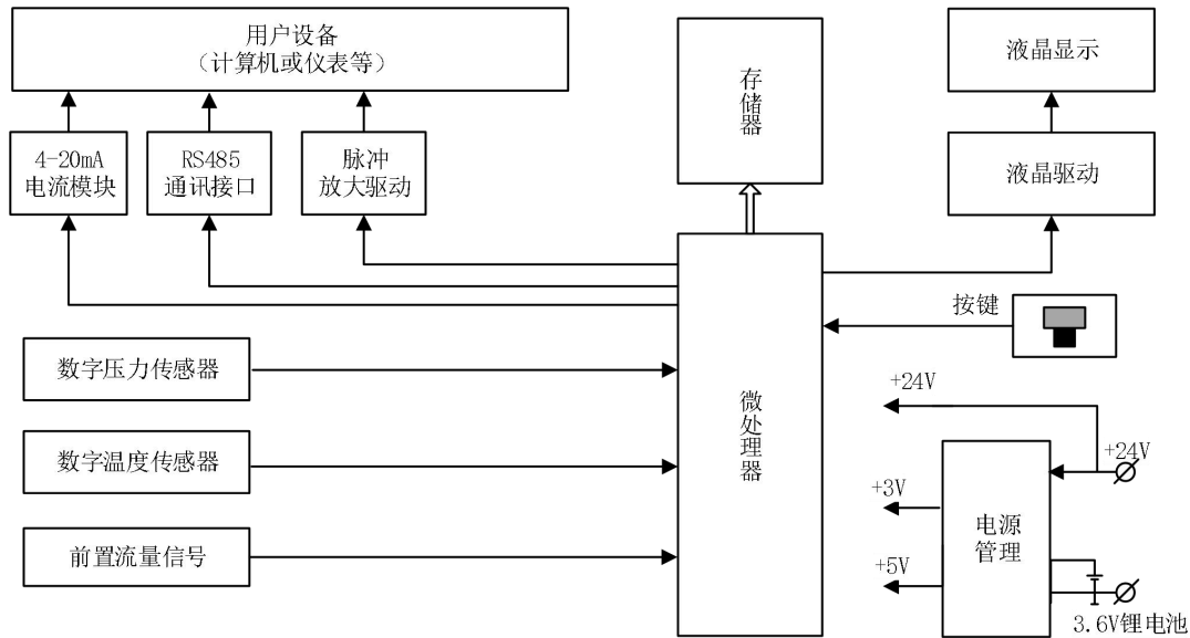
图 2 流量积算仪原理框图
