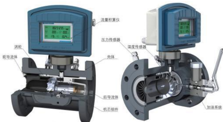
图 1 流量计原理结构图
