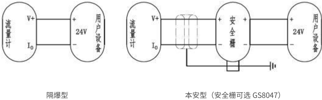
图 12-4 两线制 4 ~ 20mA 输出接线图
