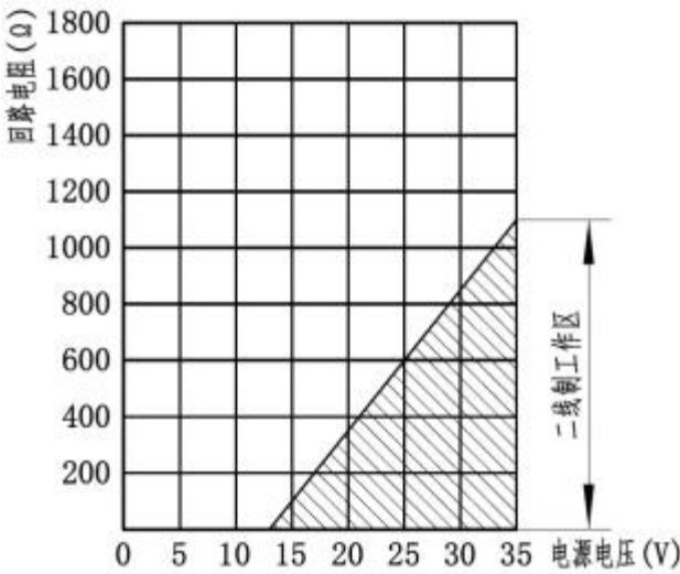
图 13 电源电压与回路电阻关系图
