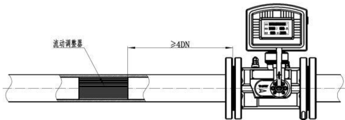
图 8 超强扰动时流量调整器安装图
