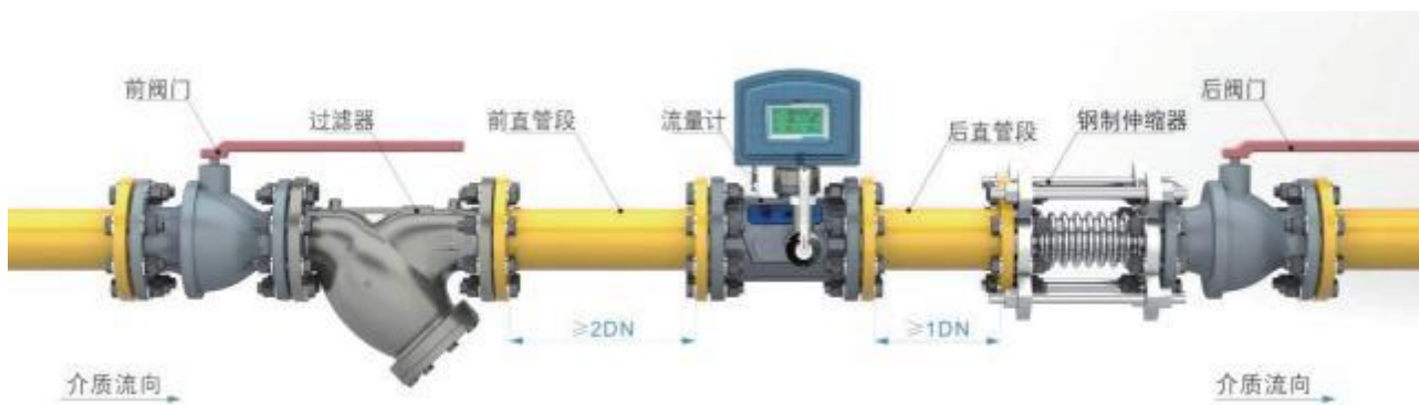
图 7 流量计水平安装示意图
