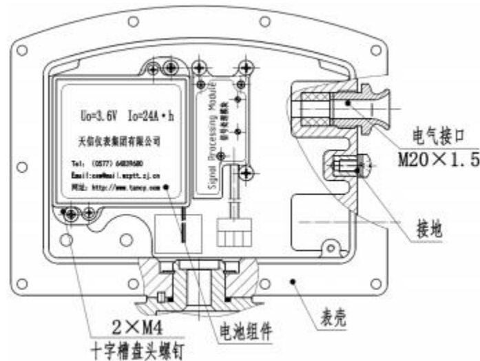
图 14 电池拆装示意图
