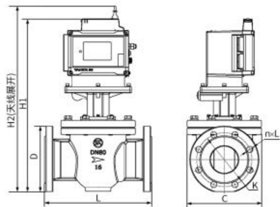
图 2-3 TCC-H 外型尺寸图
