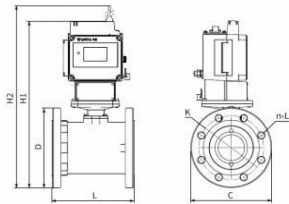
图 2-1 TCC-L 外型尺寸图
