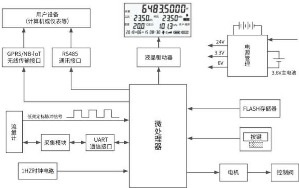
图 1 控制器原理框图
