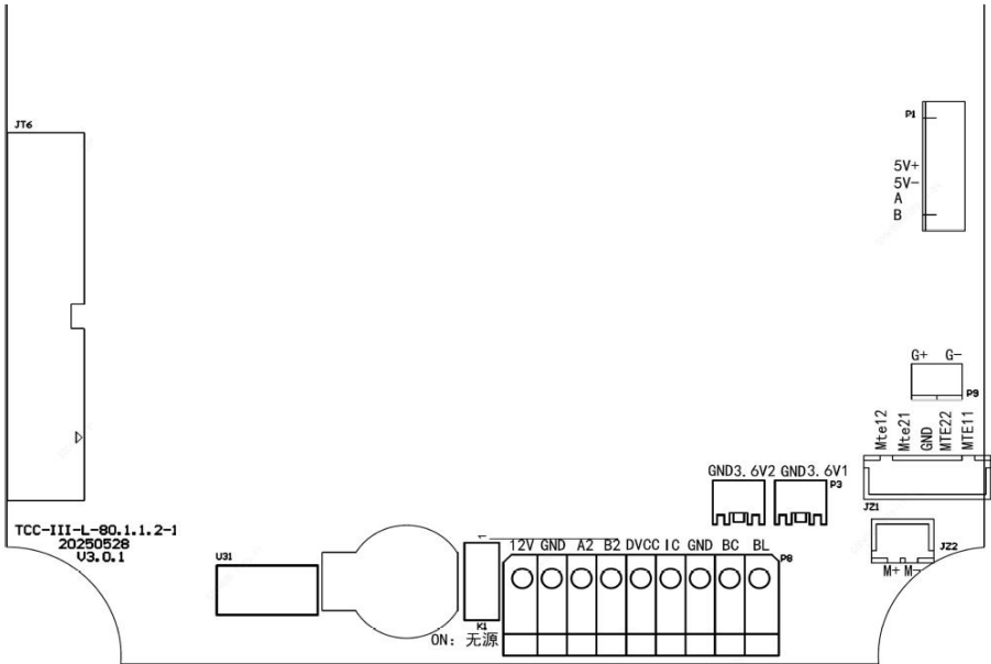
图 10-1 TCS-L 内部系统接线
