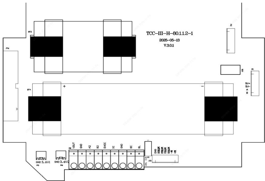
图 10-2 TCS-H 内部系统接线
