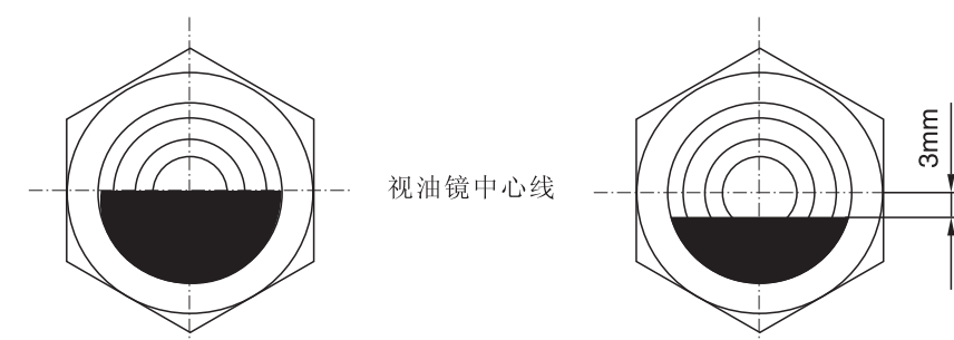
图9 视油镜油位图
