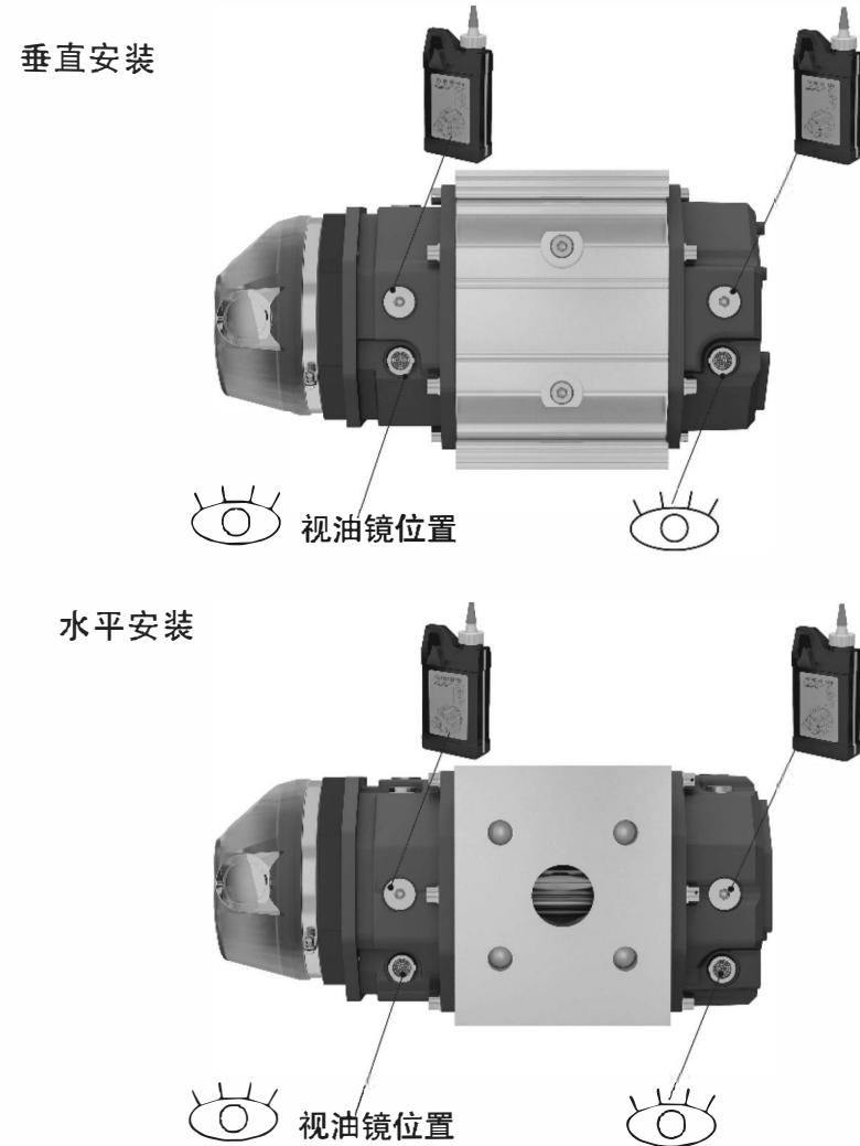
图10 注油口和视油镜位置图
