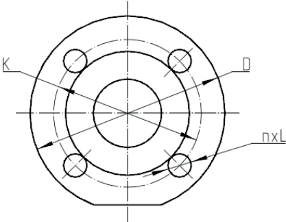
图6-1 法兰连接尺寸图
