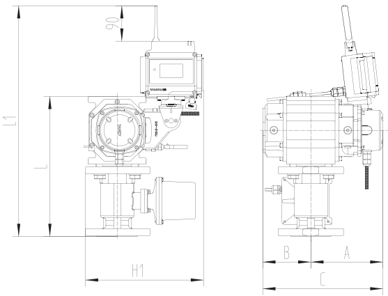
图5-6 TRMZ-G□-E/TCVL-C-E 垂直安装
