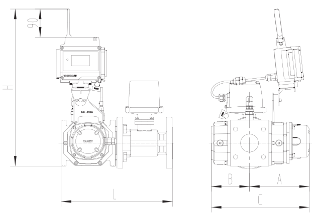
图5-5 TRMZ-G□-E/TCVL-C-E 水平安装
