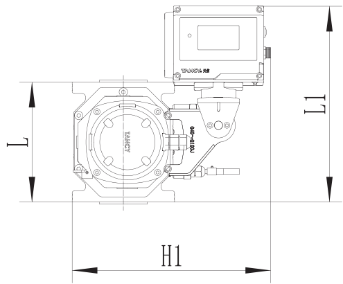
图5-2 TRMZ-G□-V 垂直安装
