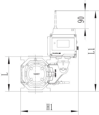
图5-4 TRMZ-G□-N、TRMZ-G□-E 垂直安装
