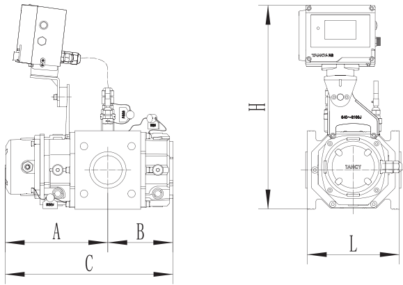
图5-1 TRMZ-G□-V 水平安装
