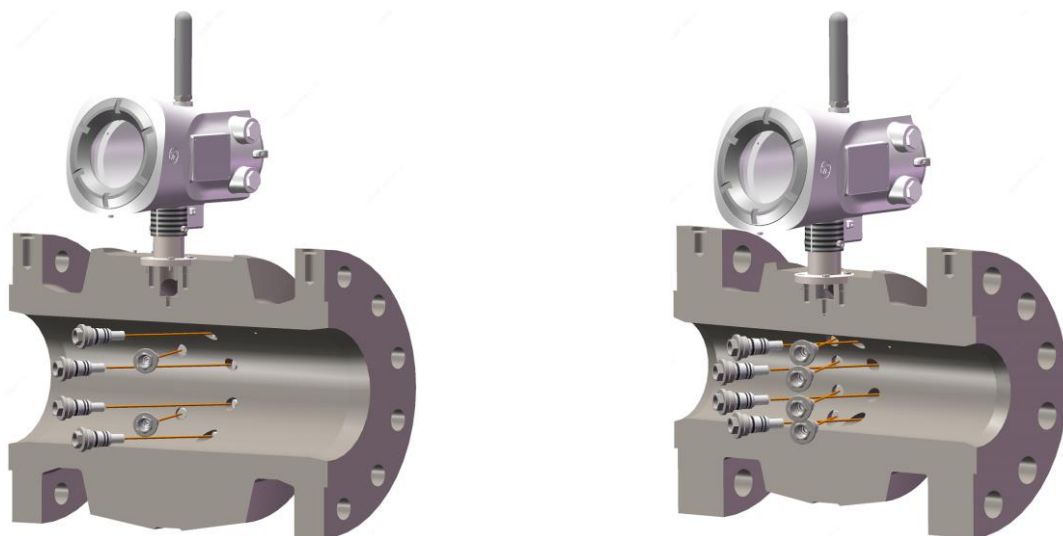
TUS-6 DN150 及以上：非对称交叉对射式六声道
