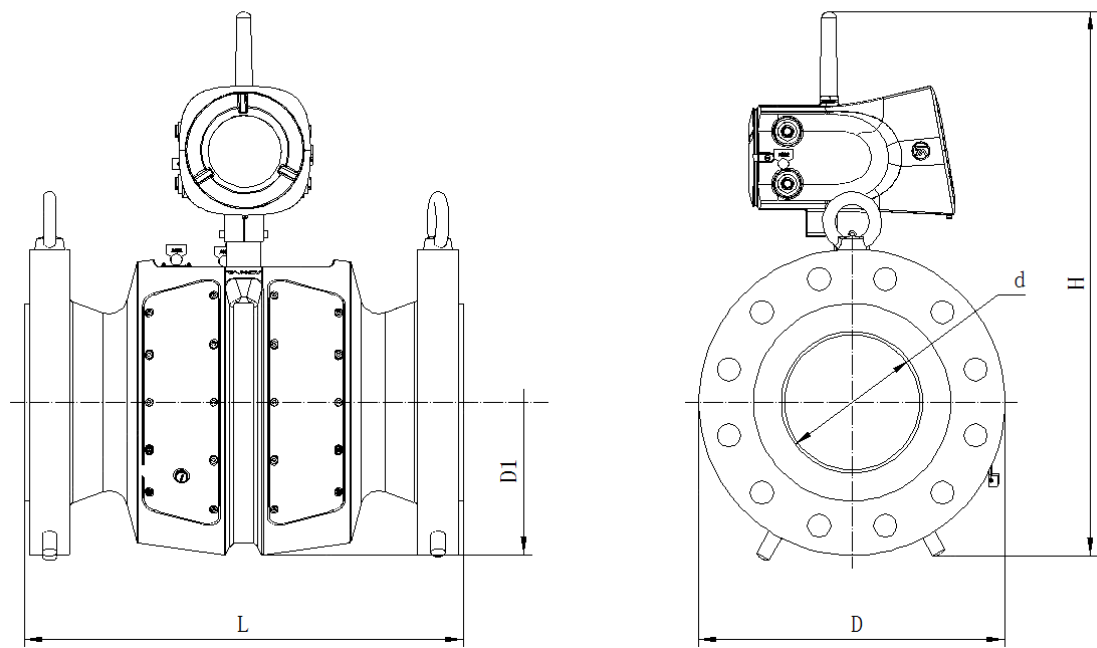
图 4 外形尺寸
