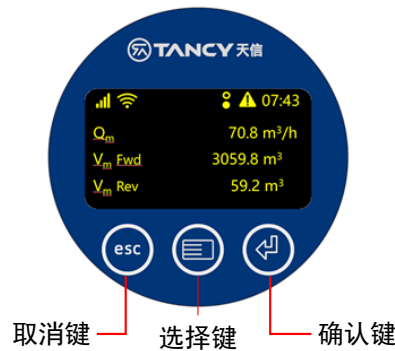
图 7 用户界面
