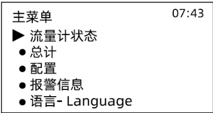
图 9 主菜单
