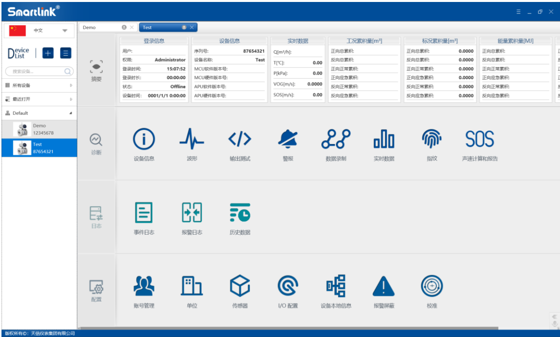
图 14 SmartLink ® 软件
