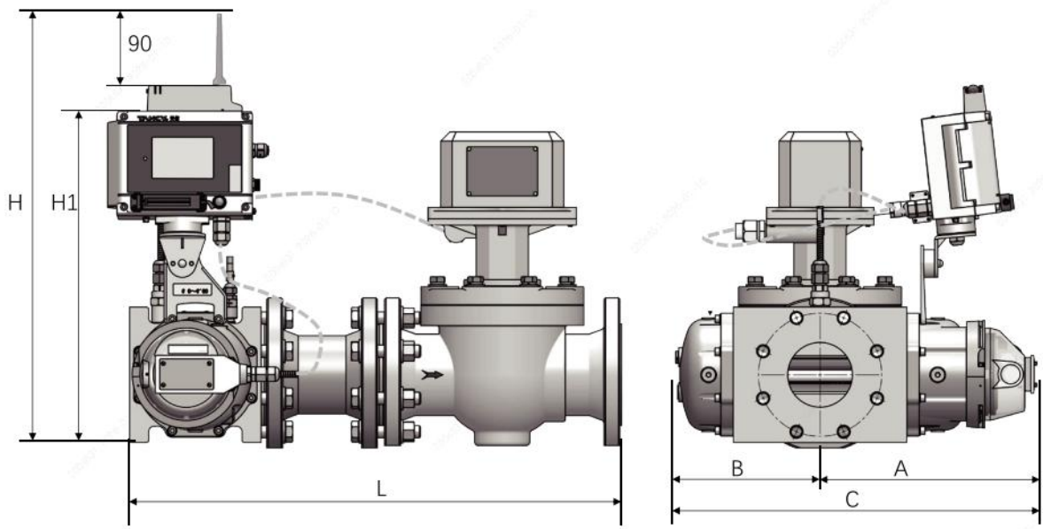
图 5-6 TYL-G□/ FCC-□-B 水平安装
