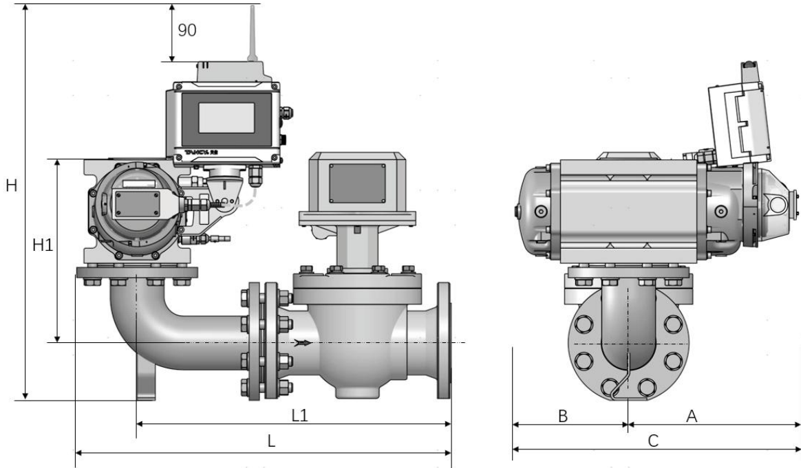
图 5-14 TYL-G□/TFC-B/TCVL-B-□-R 垂直安装
