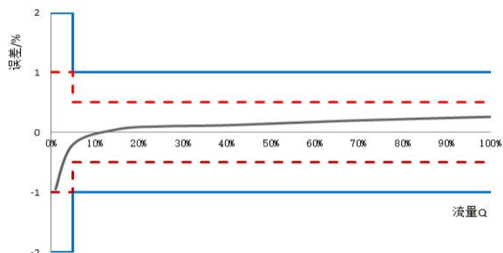
图3 典型误差特性曲线图
