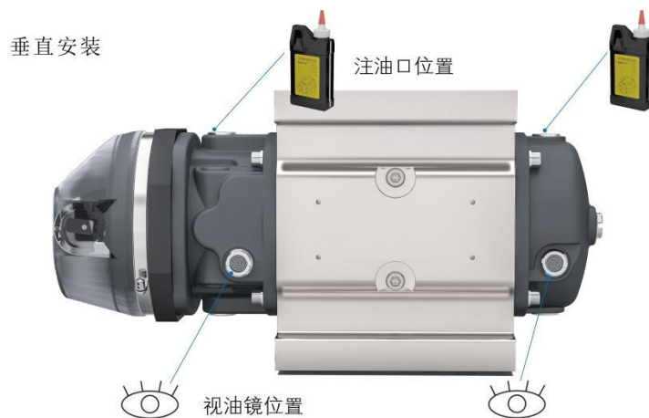
图9 视油镜油位图
