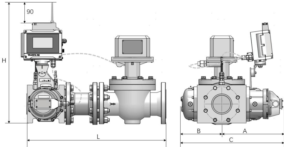
图 5-13 TYL-G□/TFC-B/TCVL-B-□-R 水平安装
