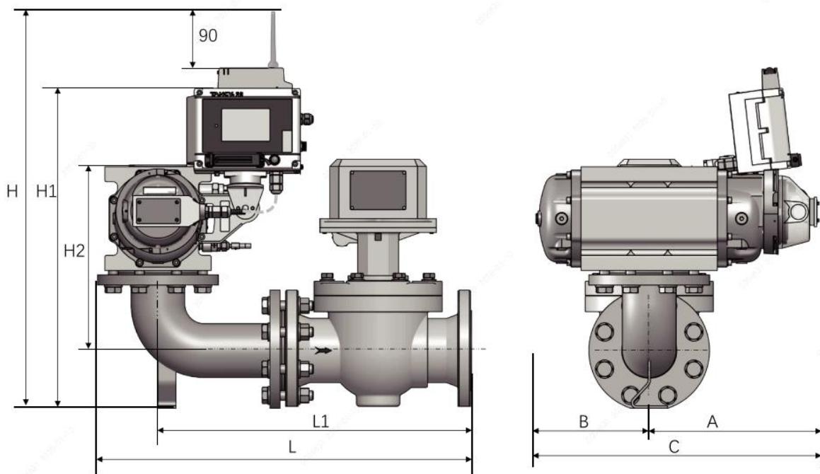
图 5-7 TYL-G□/FCC-□-B 垂直安装
