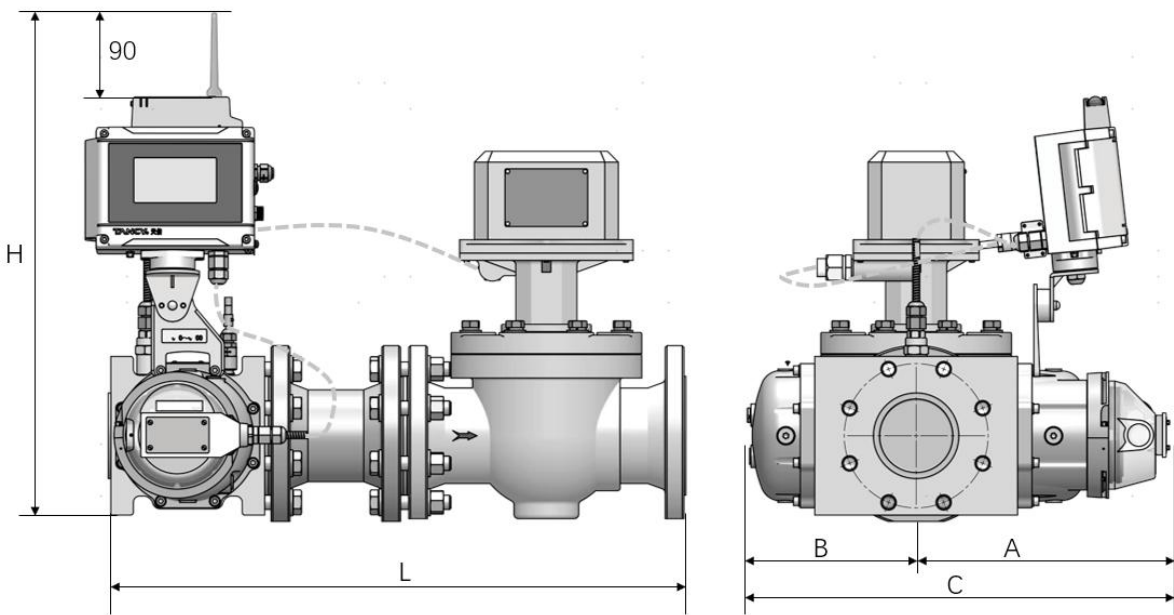
图 5-16 TYL-G□/TFC-B/TCVL-M-□-R(DN150、DN200)水平安装
