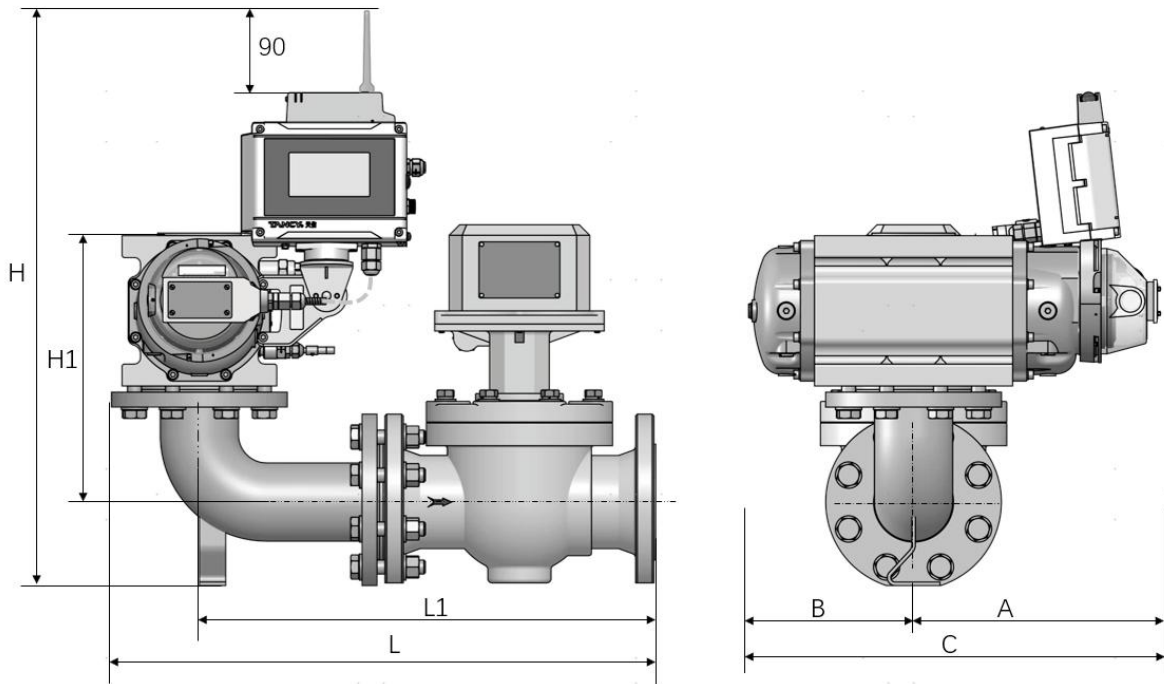
图 5-17 TYL-G□/TFC-B/TCVL-M-□-R(DN150、DN200)垂直安装
