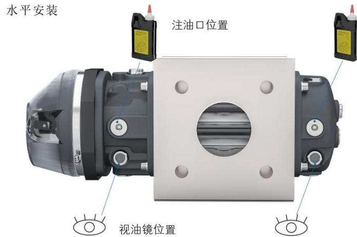
图 10-1 G6~G400-4 注油口和视油镜位置图
