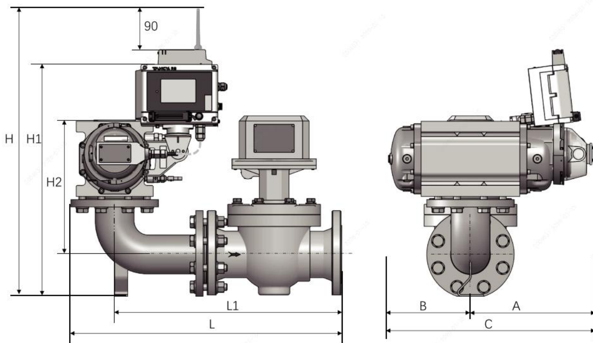
图 5-10 TYL-G□/ FCC-□-M(DN150、DN200)垂直安装
