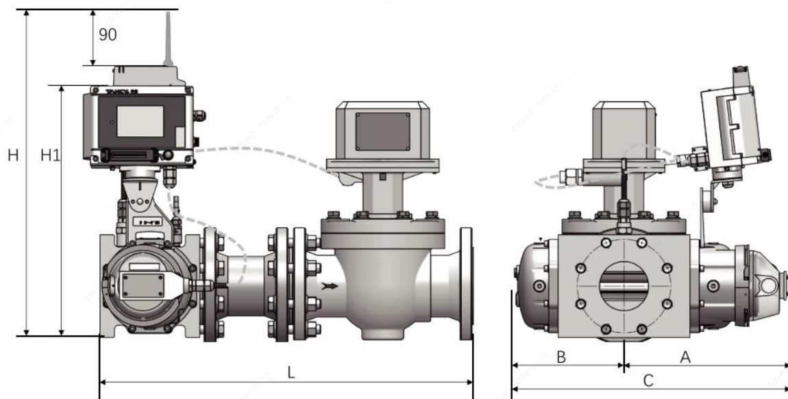
图 5-9 TYL-G□/ FCC-□-M(DN150、DN200)水平安装
