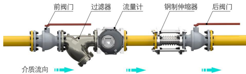
图 8 水平安装示意图
