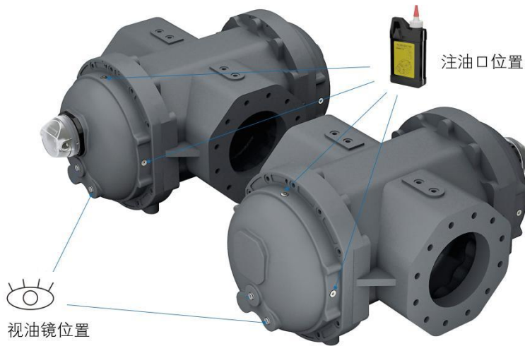
图 10-2 G400-6~G1000 注油口和视油镜位置图
