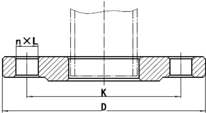
图6-2 突面（RF）板式平焊钢制管法兰
