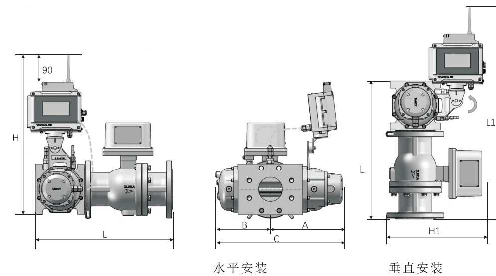
图5-12 TYLZ-G□-□/TCVL-M-□-R
