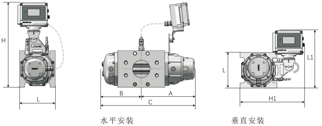
图5-3 TYLZ-G□-V
