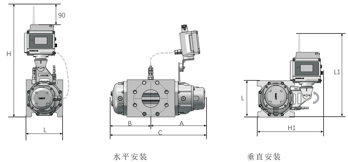
图5-4 TYLZ-G□-N
