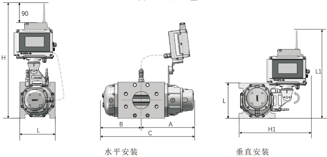
图5-1 TYLZ-G□
