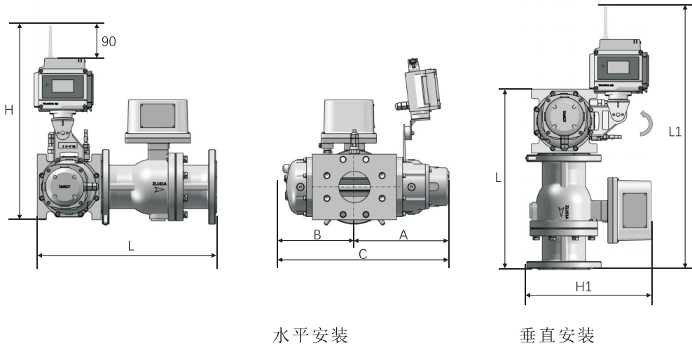
图5-9 TEP-G□-1-M
