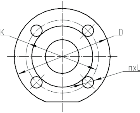
图6-3 法兰连接尺寸图
