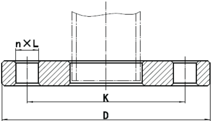
图6-1 平面（FF）板式平焊钢制管法兰
