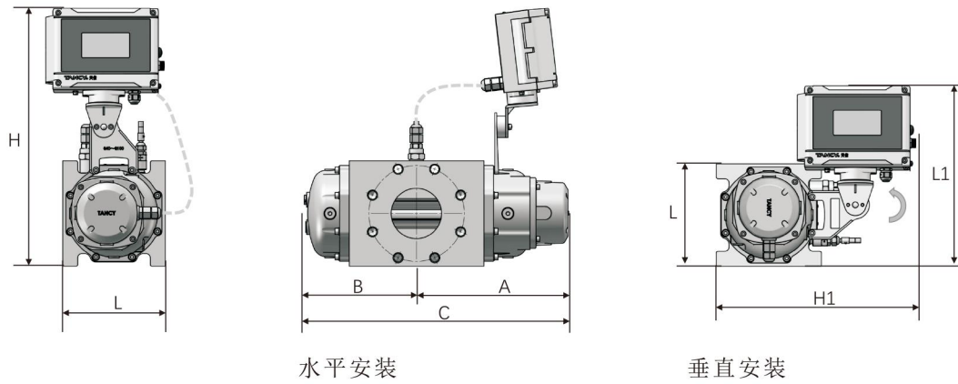
图5-1 TYLZ-G□
