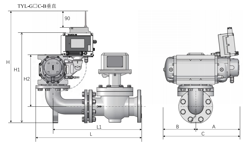
图5-6 TYL-G□C-B垂直安装
